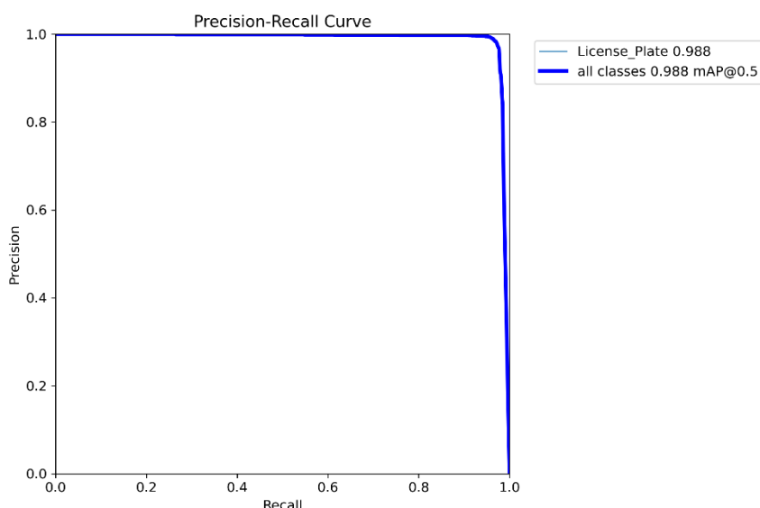
Slika 19. Preciznost - Prisjećanje krivulja na modelu treniranom za detekciju registrarskih pločica
