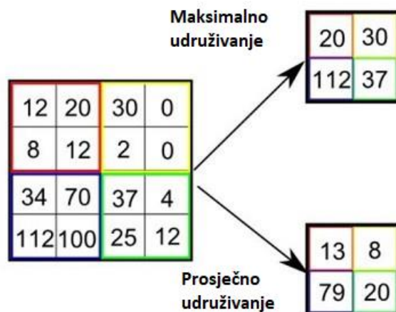
Slika 15. Maksimalno i prosječno udruživanje s iskorakom 2 i 2×2 filterom
