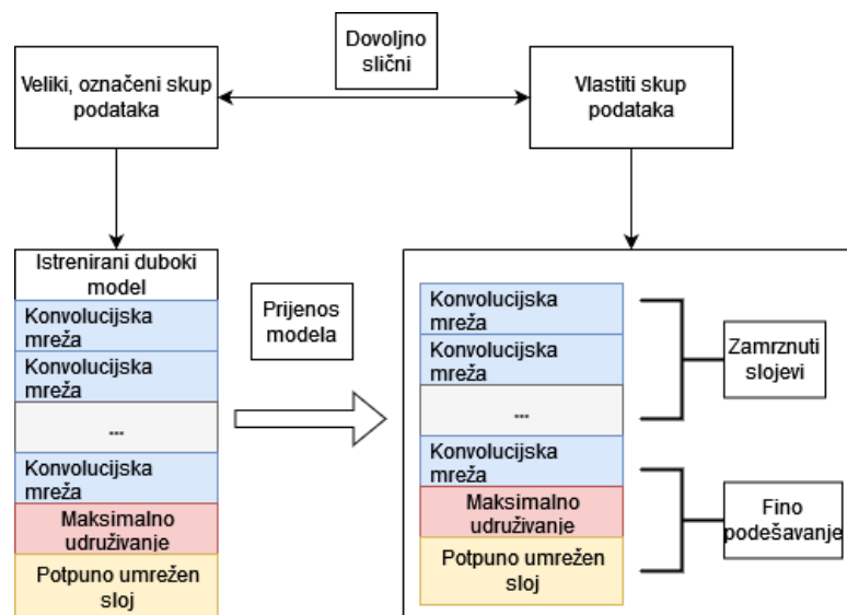
Slika 18. Prijenosno učenje
