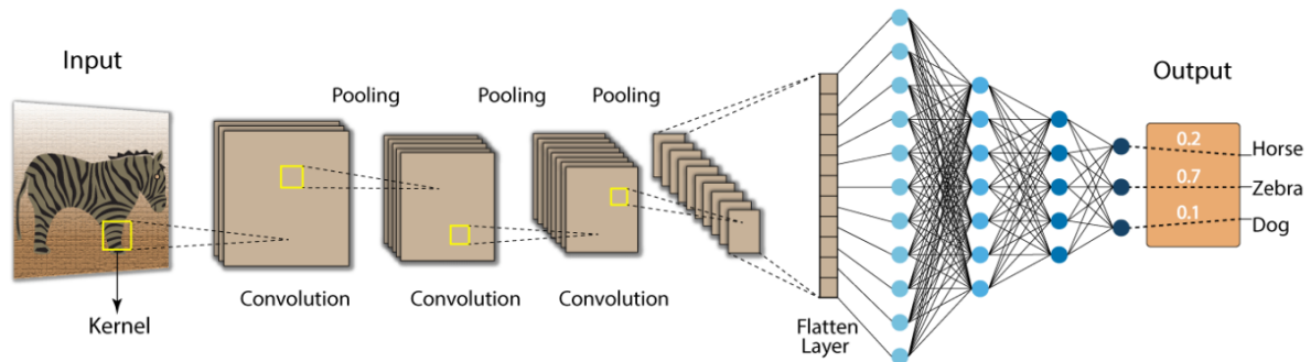
Slika 4. CNN proces [15]
