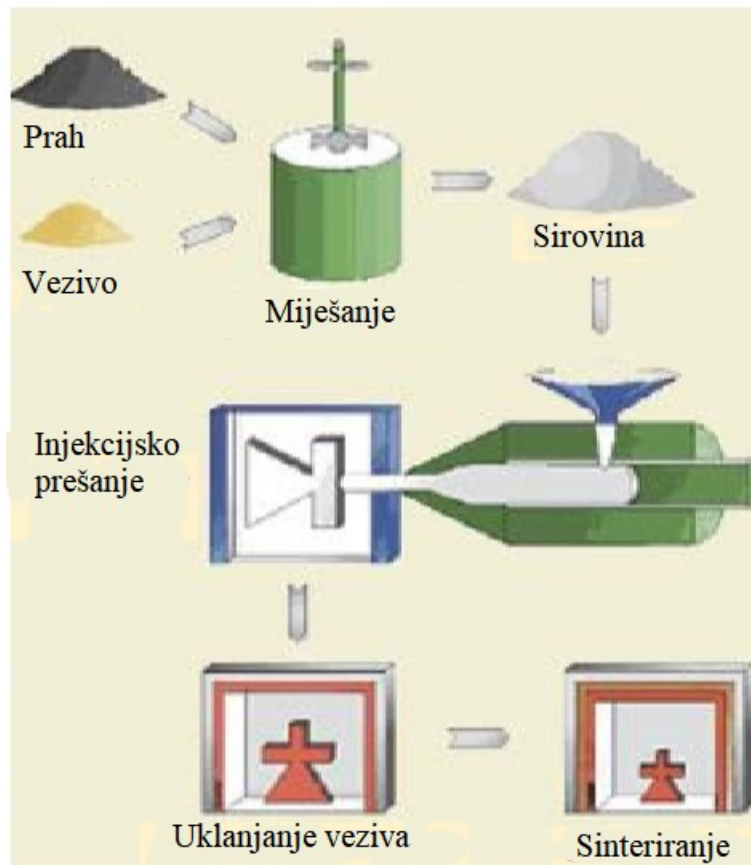
Slika 2. Postupak injekcijskog prešanja metala [3]
