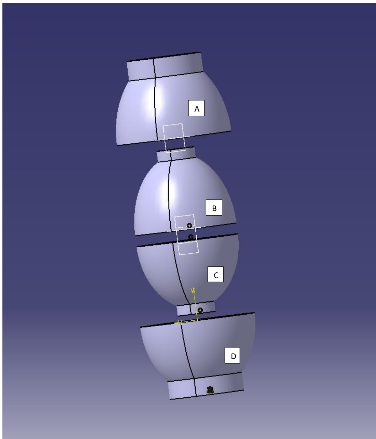
Slika 21. Rastavljeni prikaz
