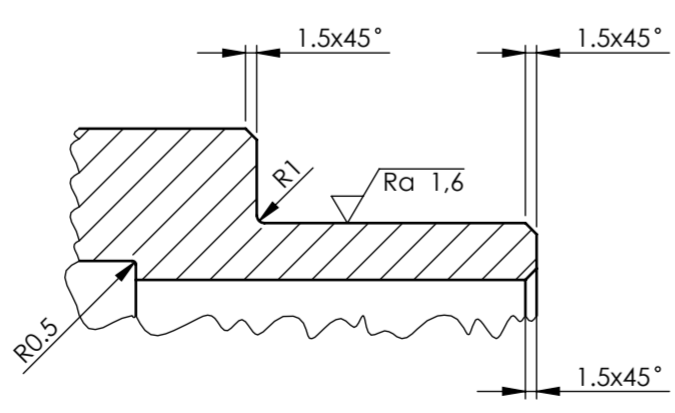
Detalj C (Mjerilo 1 : 1)
