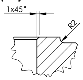
Detalj D (Mjerilo 1 : 1)
