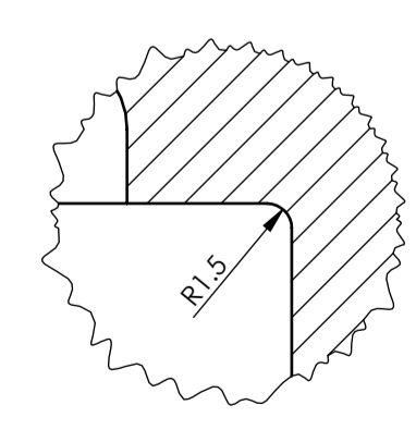
Detalj H (Mjerilo 2 : 1)
