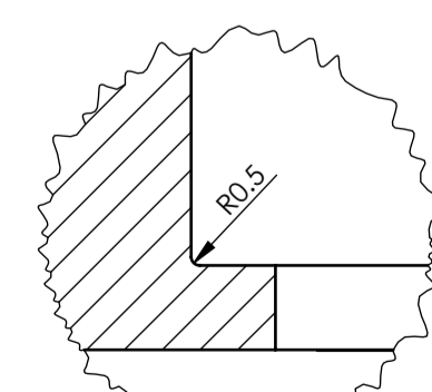
Detalj G (Mjerilo 2 : 1)
