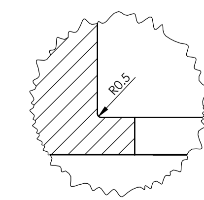
Detalj G (Mjerilo 2 : 1)
