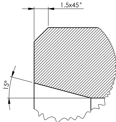
Detalj B (Mjerilo 5 : 1)
