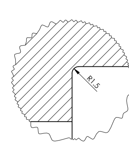
Detalj E (Mjerilo 2 : 1)
