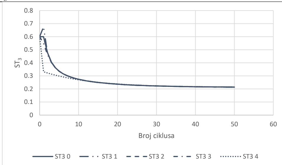
Dijagram 5.26, ST stroja 3 račun analičkom metodom za slučaj B
