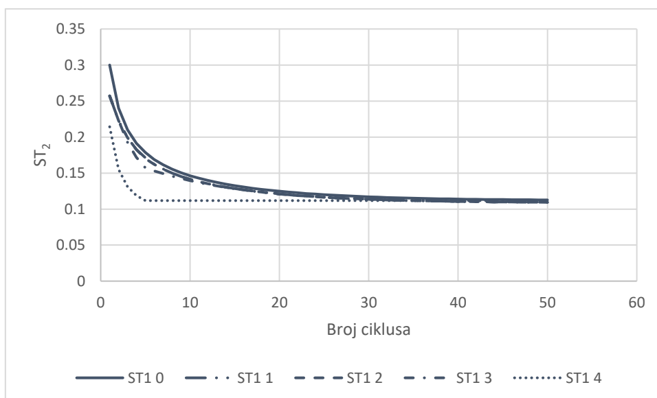
Dijagram 5.27, ST stroja 2 račun metodom konačnih stanja za slučaj B
