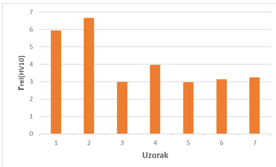
Slika 25. Dijagram nejednolikosti površinske tvrdoće za metodu HV10
