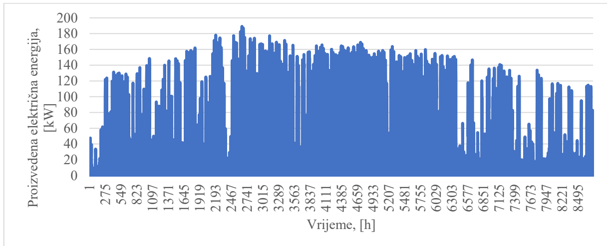
Slika 34. Električna energija generirana transparentnim solarnom panelima
