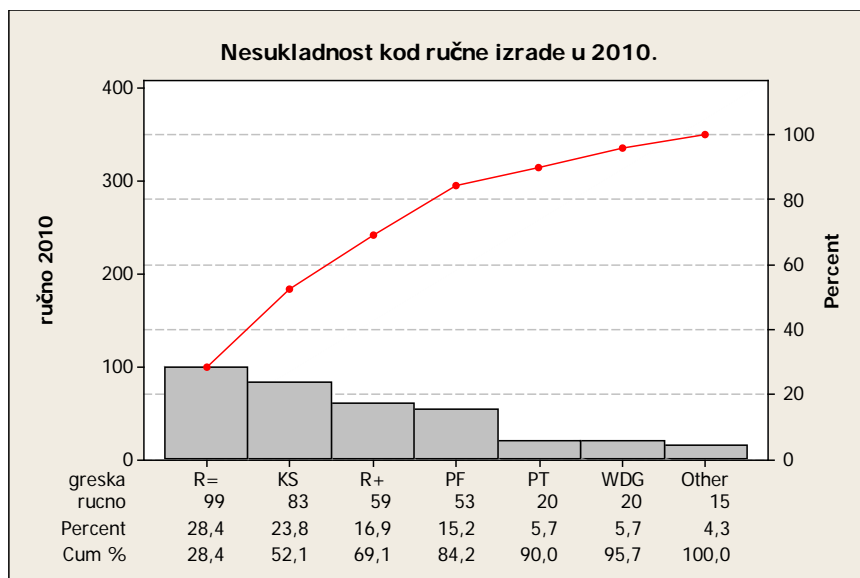
Dijagram 5.4 Pareto dijagram nesukladnosti u 2010. godini kod ručnog namatanja u namatonici
