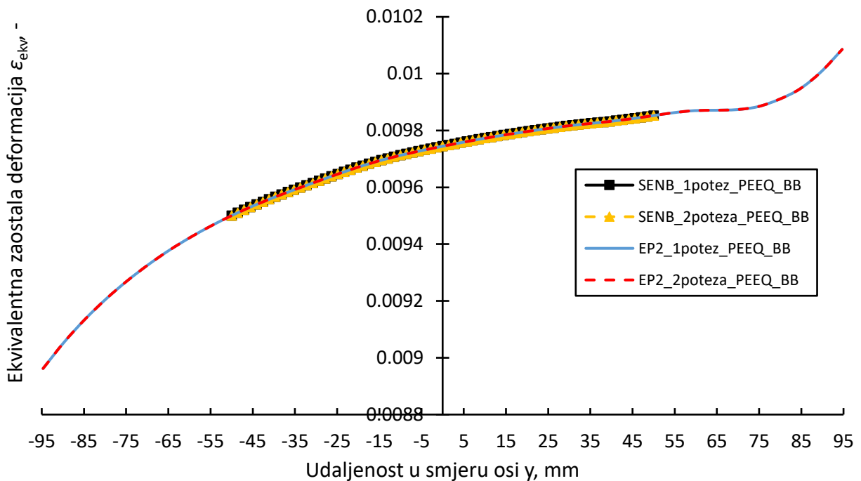
Slika 69 Dijagram zaostalih ekvivalentnih deformacija \varepsilon_{ekv} longitudinalnih epruveta na presjeku B-B
