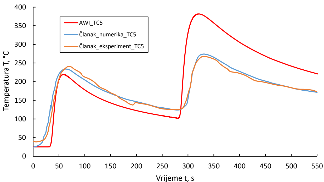
Slika 21 Promjena temperature kroz vrijeme u točki TC5
