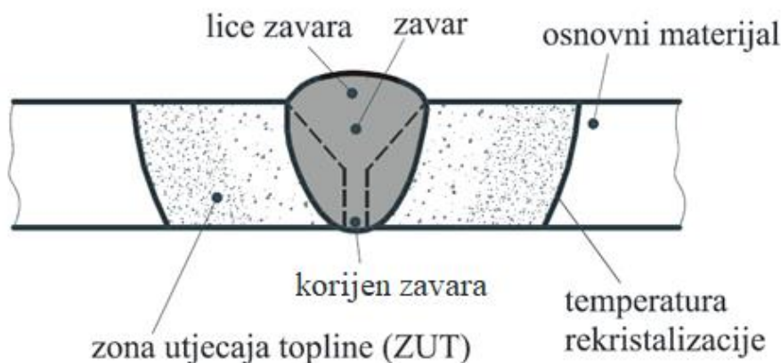
Slika 1 Sučeoni zavar [5]
