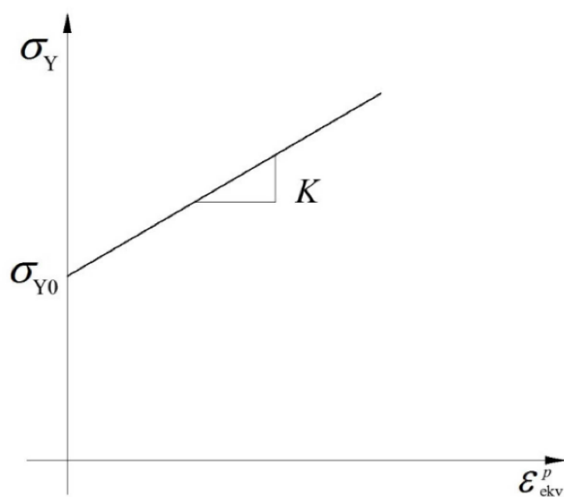
Slika 6 Linearno očvršćenje [12]
