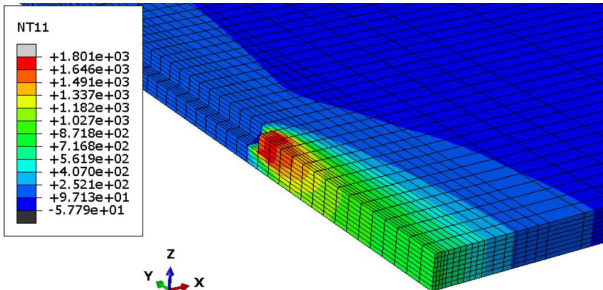
Slika 19 Temperaturno polje 3D modela u 265. sekundi toplinske analize
