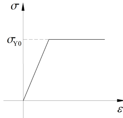
Slika 3 Dijagram naprežanja i deformacija elastično-idealno plastičnog materijala [12]
