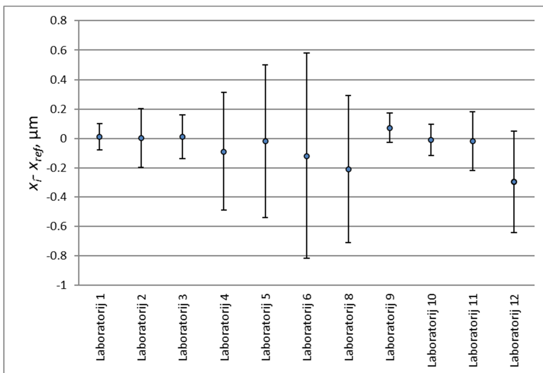
Slika 15. Prikaz odstupanja laboratorija od referentne vrijednosti u EURAMET L-K4 usporedbi nakon izbacivanja Laboratorija 7 iz usporedbe za nazivni promjer \varnothing 5 mm u slučaju referentne vrijednosti određene aritmetičkom srednjom vrijednosti
