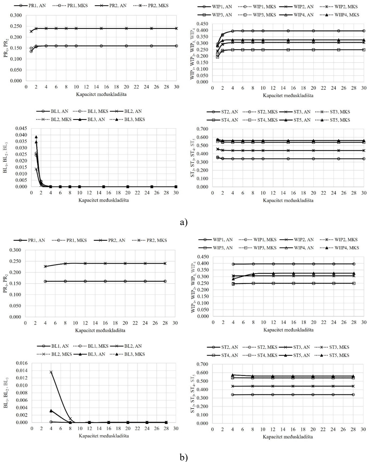
Slika 4.11 Usporedba ključnih značajki, a) linija L5D, N_1=N_2=N_3=N_4=N , b) linija L5D, N_1=N , N_2=3/4N , N_3=1/2N , N_4=1/4N [77]
