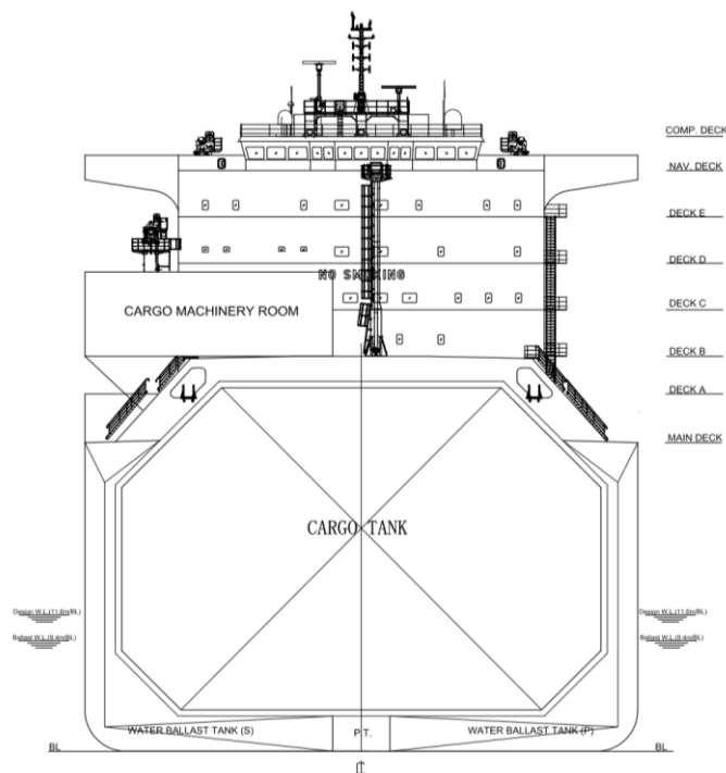
Slika 3-1 Poprečni presjek broda
