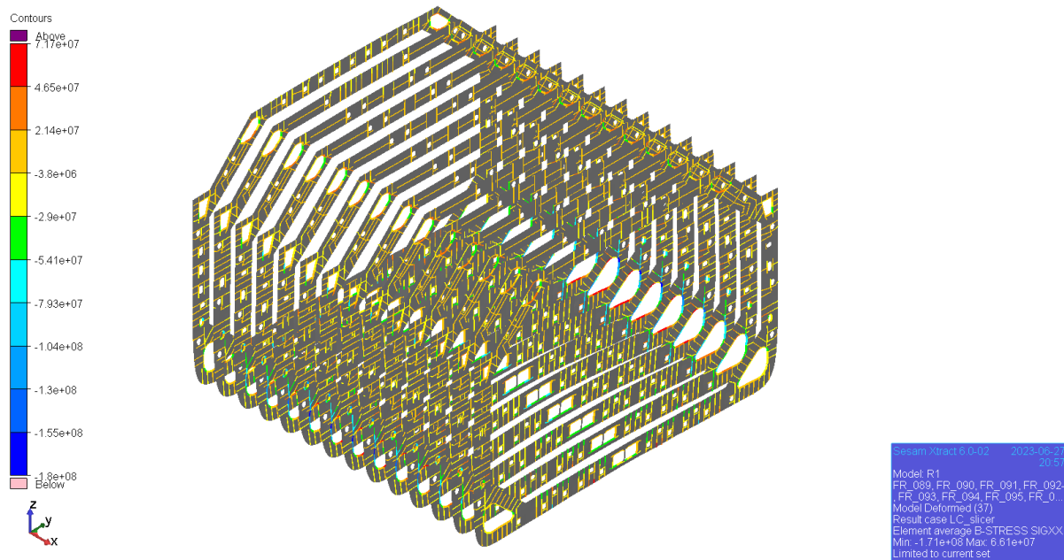
Slika 6-19 Aksijalna napreznja u grednim konačnim elementima na okvirnim rebrima [Pa]
