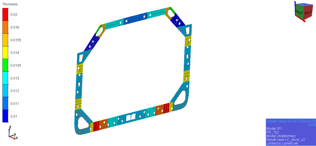
Slika- B-III Debljine na tipičnom rebru [m]
