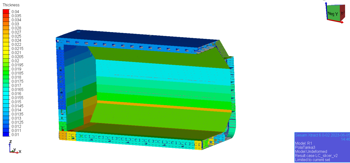
Slika- B-IV Debljine unutar srednjeg skladišta [m]
