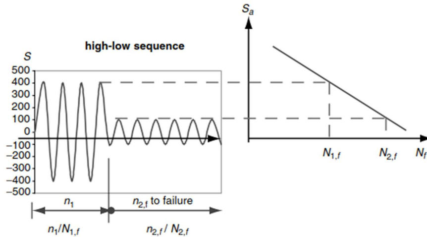
Slika 7-1 Odnos između broja ciklusa naprezanja i vijeka trajanja konstrukcije pod tim napreznjima [29]
