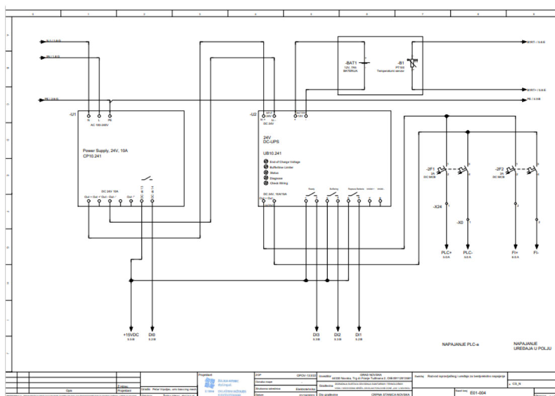
Slika 8: Shema upravljačkog ormarića – Stranica 3
