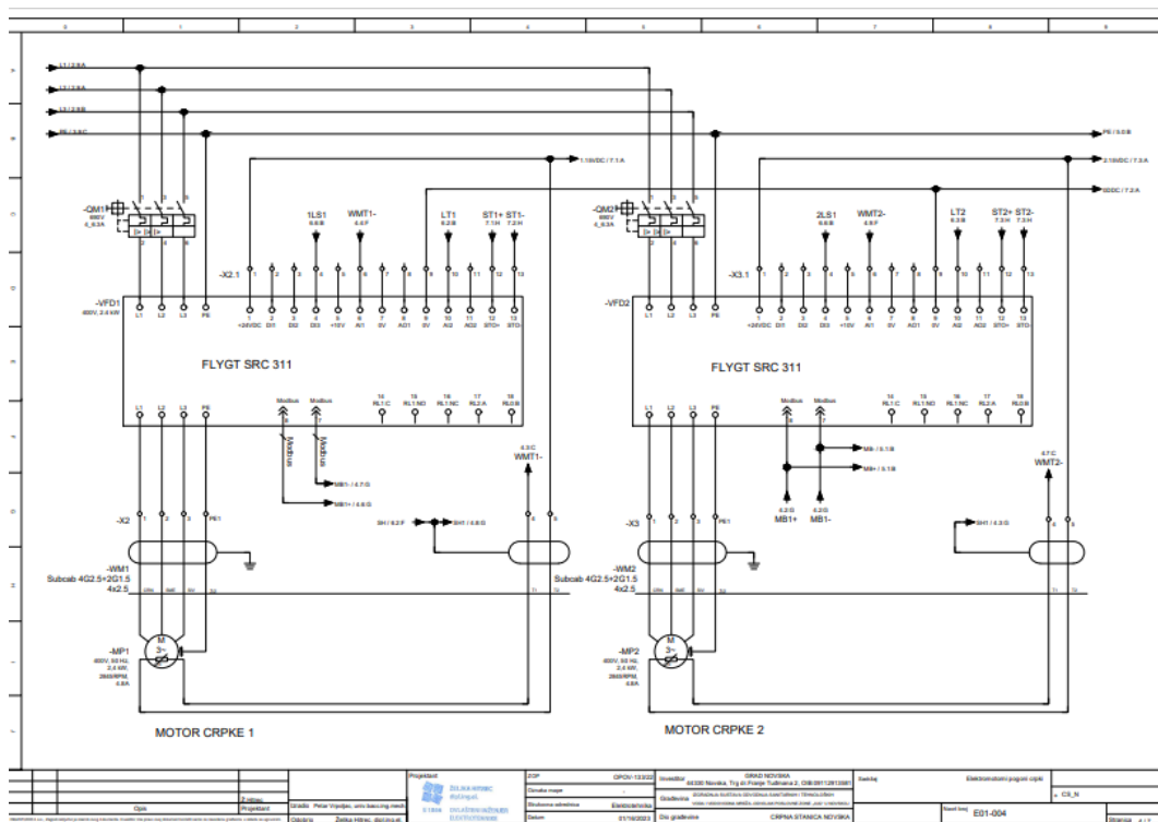
Slika 9: Shema upravljačkog ormarića – Stranica 4
