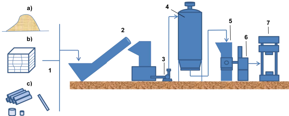
Slika 4.4. Postrojenje za pravljenje izravno prešanih otpresaka od otpadne plastike a - granulirani smećci, b - kompoziti, filmovi, folije, runo, c - kruta plastika, 1 - plastični otpad, 2 - usitnjavalica, 3 - mehanička ili pneumatska dobava, 4 - silo, 5 - plastifikator s istiskivalicom, 6 - volumno doziranje (obujmena odmjera) plastifikata, 7 - automatska dobava preša za izravno prešanje [1]
