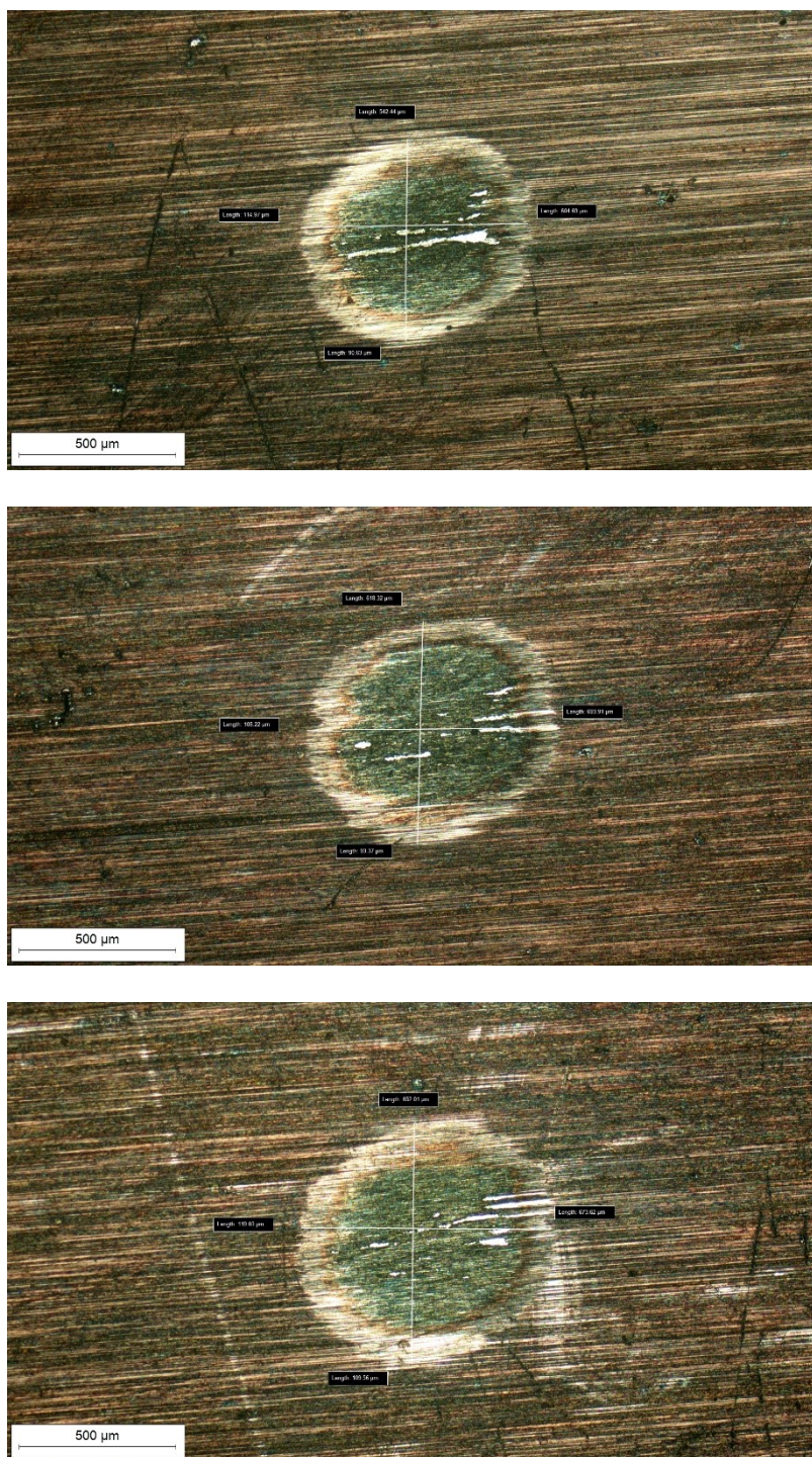
Slika 32. Prikaz otisaka dobivenih kalotestom na uzorku A2
