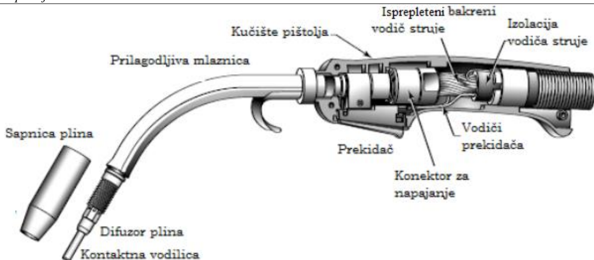
Slika 2. Pištolj za zavarivanje MIG postupkom u poprečnom presjeku [9]
