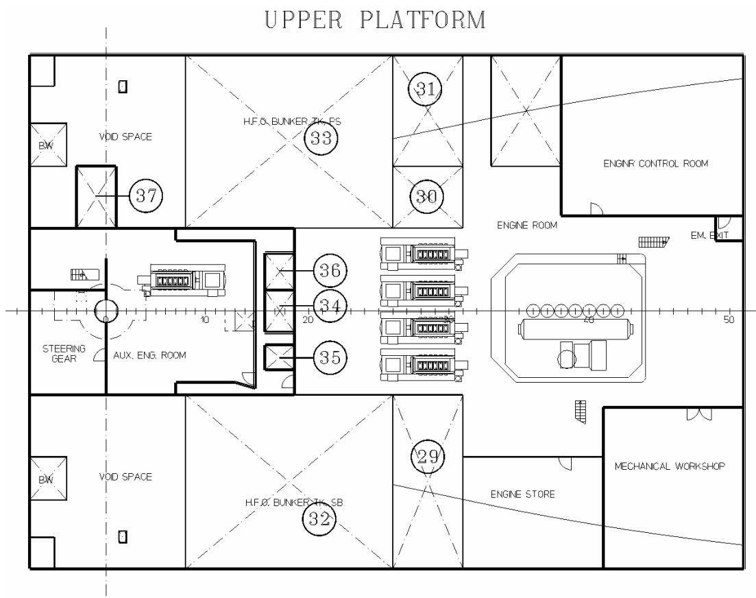
Slika 18. Prikaz strojarnice gradnje 428 – gornja platforma strojarnice
