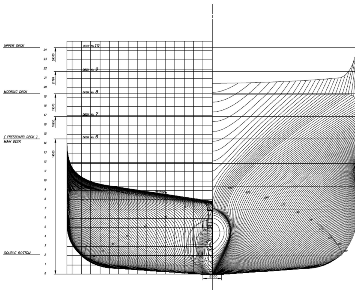
Slika 28. Poprečni presjek
