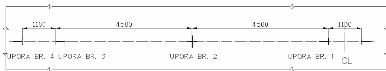
Slika 33. Raspored upora
