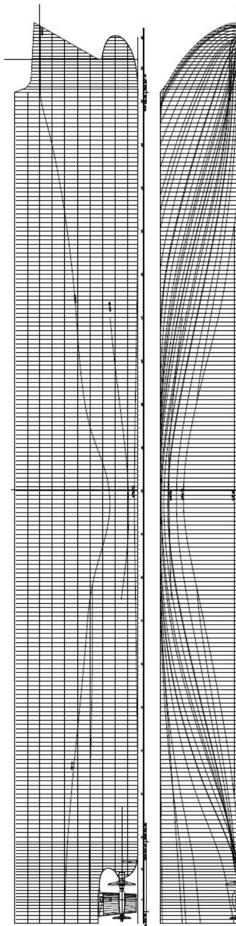
Slika 29. Uzdužni presjek
