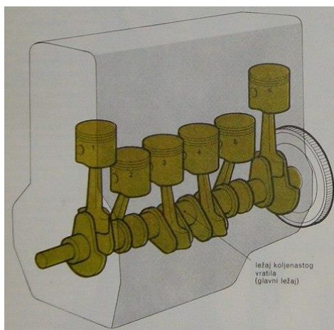
Slika 4. Redni motor [5]
