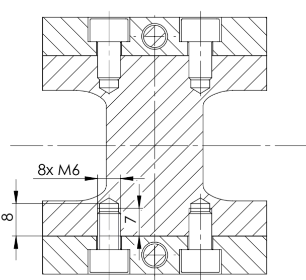
Presjek A-A
