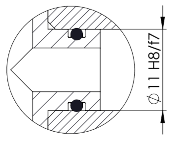
DETAIL C M 2:1
