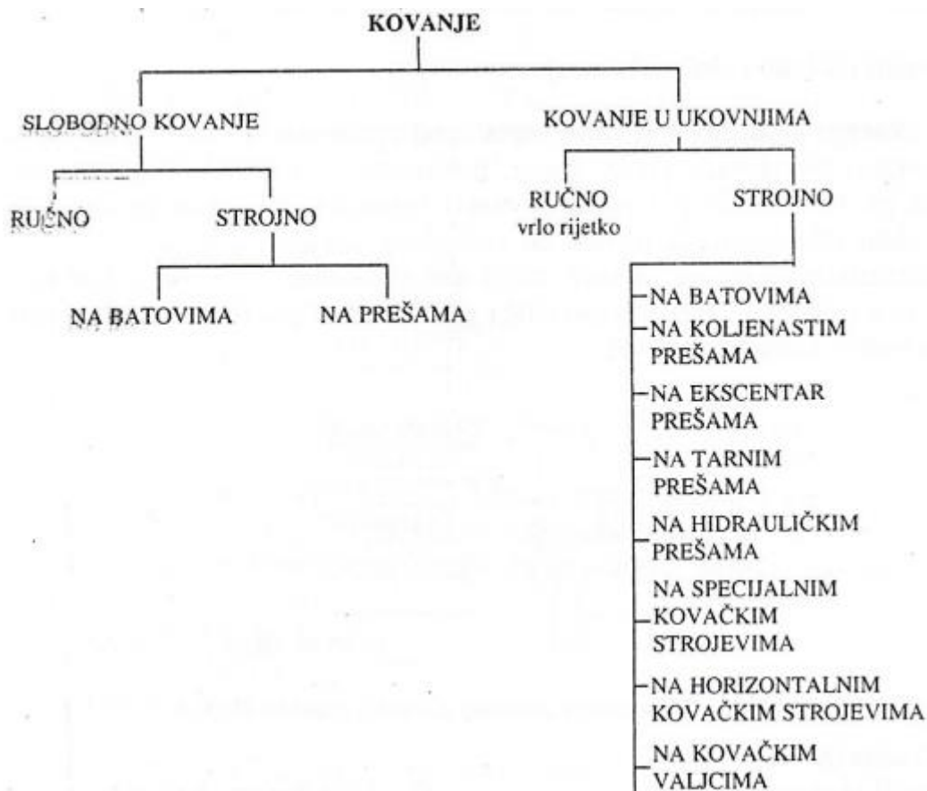
Slika 16. Podjela kovanja [15]
