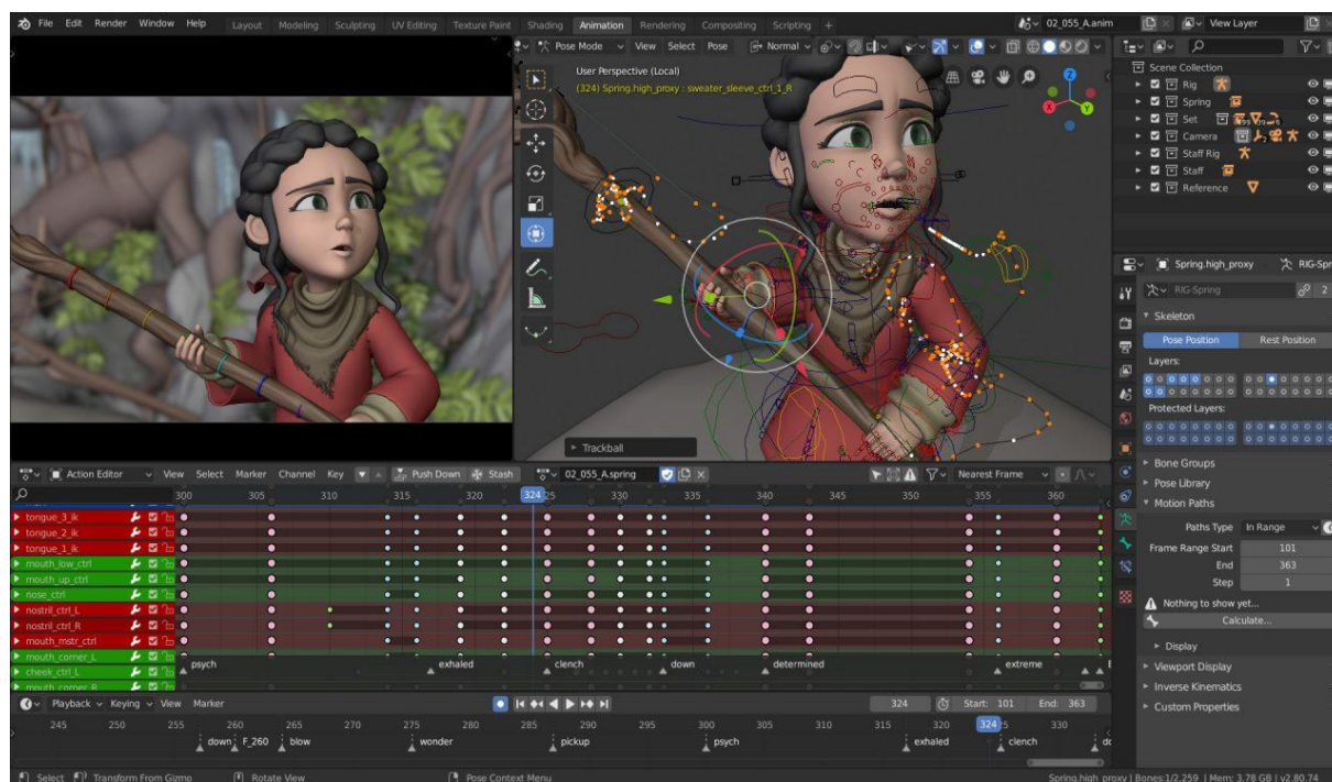
Slika 26. Softver Blender [34]
