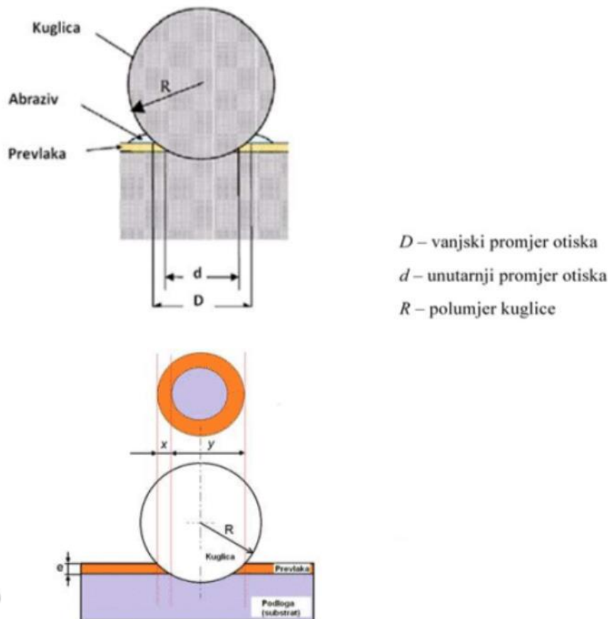
Slika 13: Kalotest, određivanje debljine prevlake [21]
