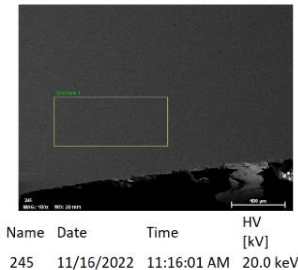
Slika 33: Područje EDX ispitivanja na tijelu glavčine
