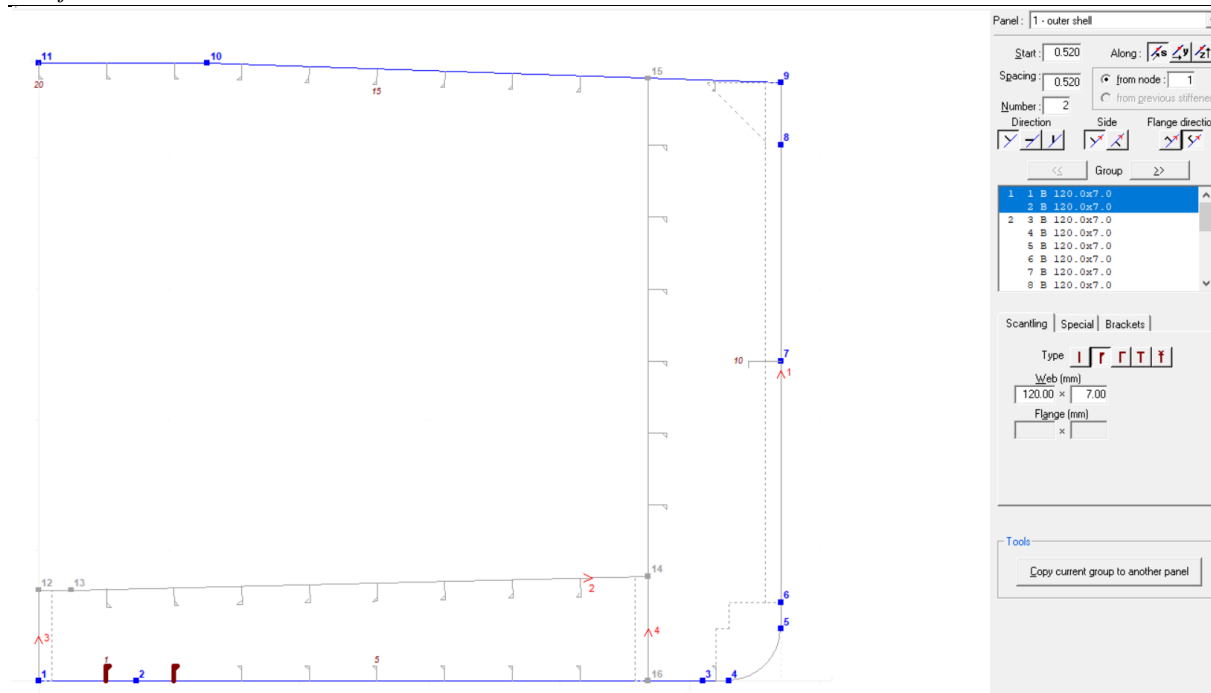
Slika 7. Generiranje uzdužnjaka
