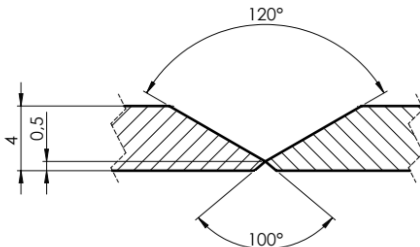
Slika 17. Priprema spoja
