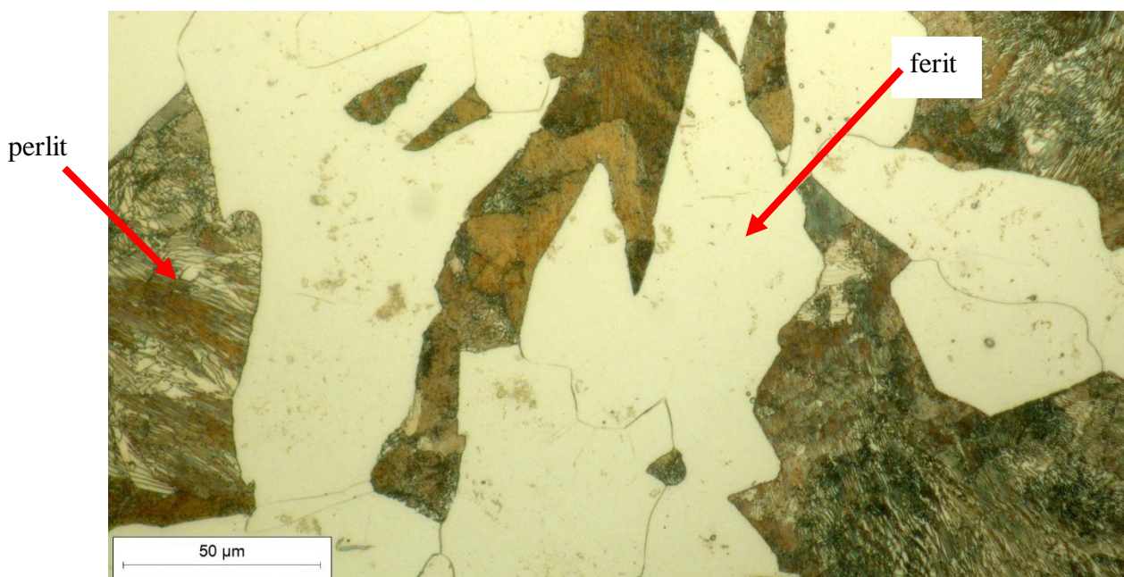
Slika 42. Mikrostruktura sredine presjeka pužnog kola, uvećana 100x
