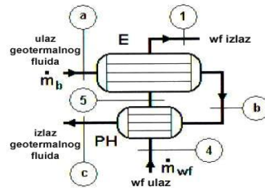
Slika 24. Predgrijač i isparivač
