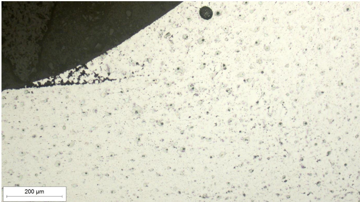
Slika 43. Mikrostruktura ZUT-a u tjemenu zavora s lijeve strane, snimljena pri povećanju 100×
