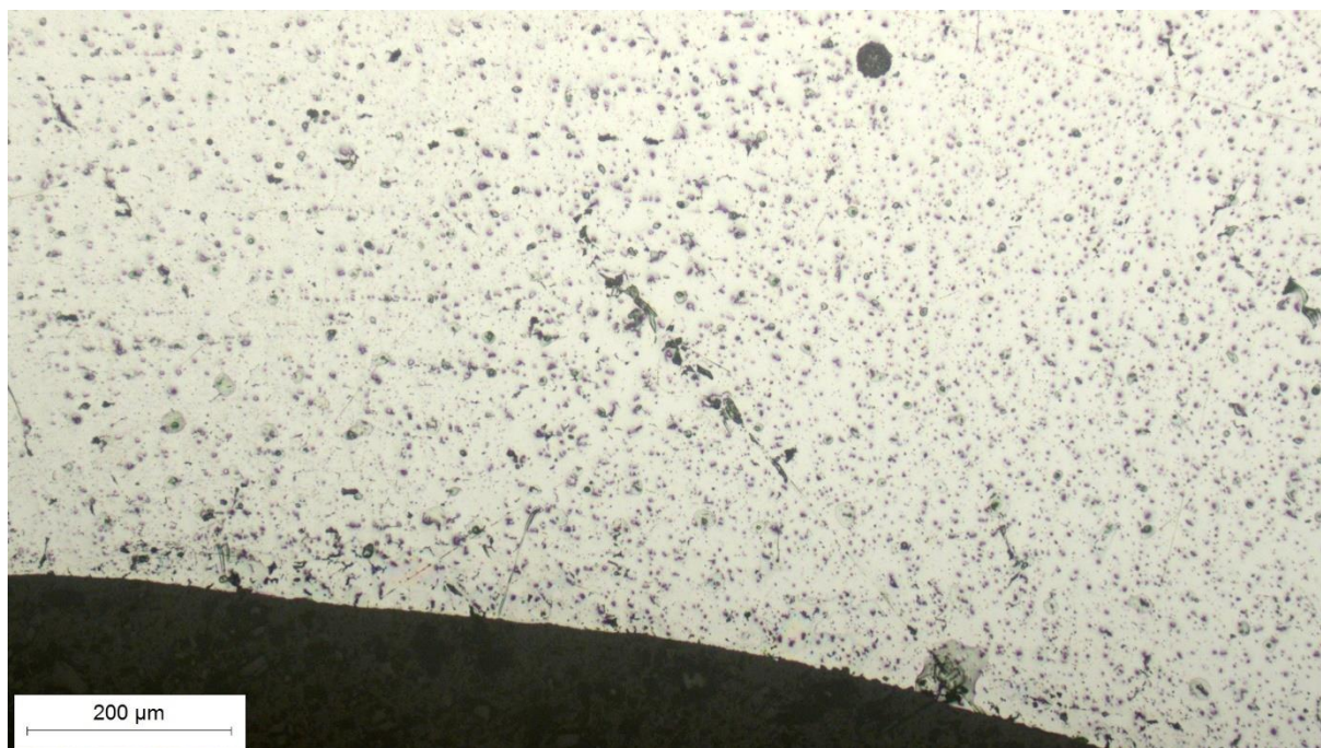
Slika 47. Mikrostruktura ZUT-a u korijenu zavarenog spoja s lijeve strane, snimljena pri povećanju od 100×
