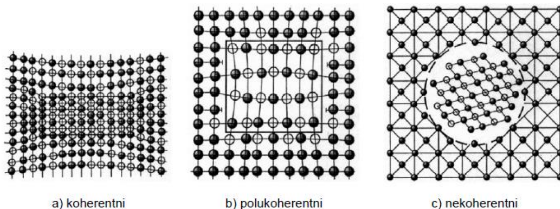
Slika 5. Tipovi precipitata [4]
