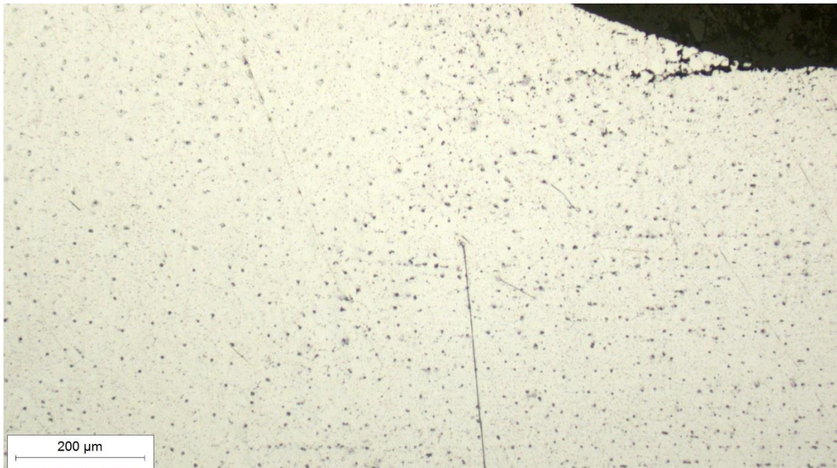
Slika 44. Mikrostruktura ZUT-a u tjemenu zavarenog spoja s desne strane, snimljena pri povećanju od 100×
