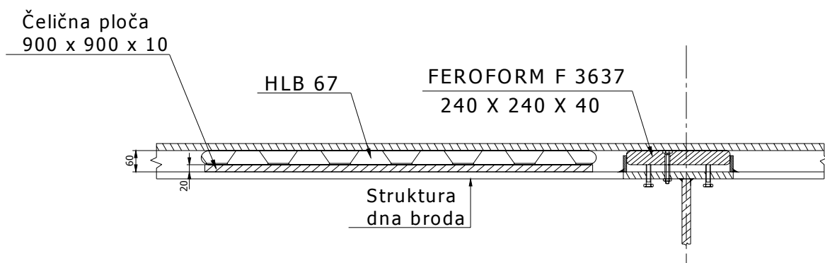
Slika 48 Konačni položaj tankova tereta oslonjenih na ploču Ferroforma
