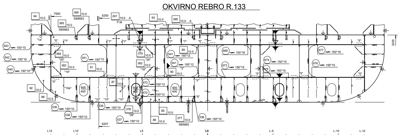
Slika 58 Okvirno rebro R133
