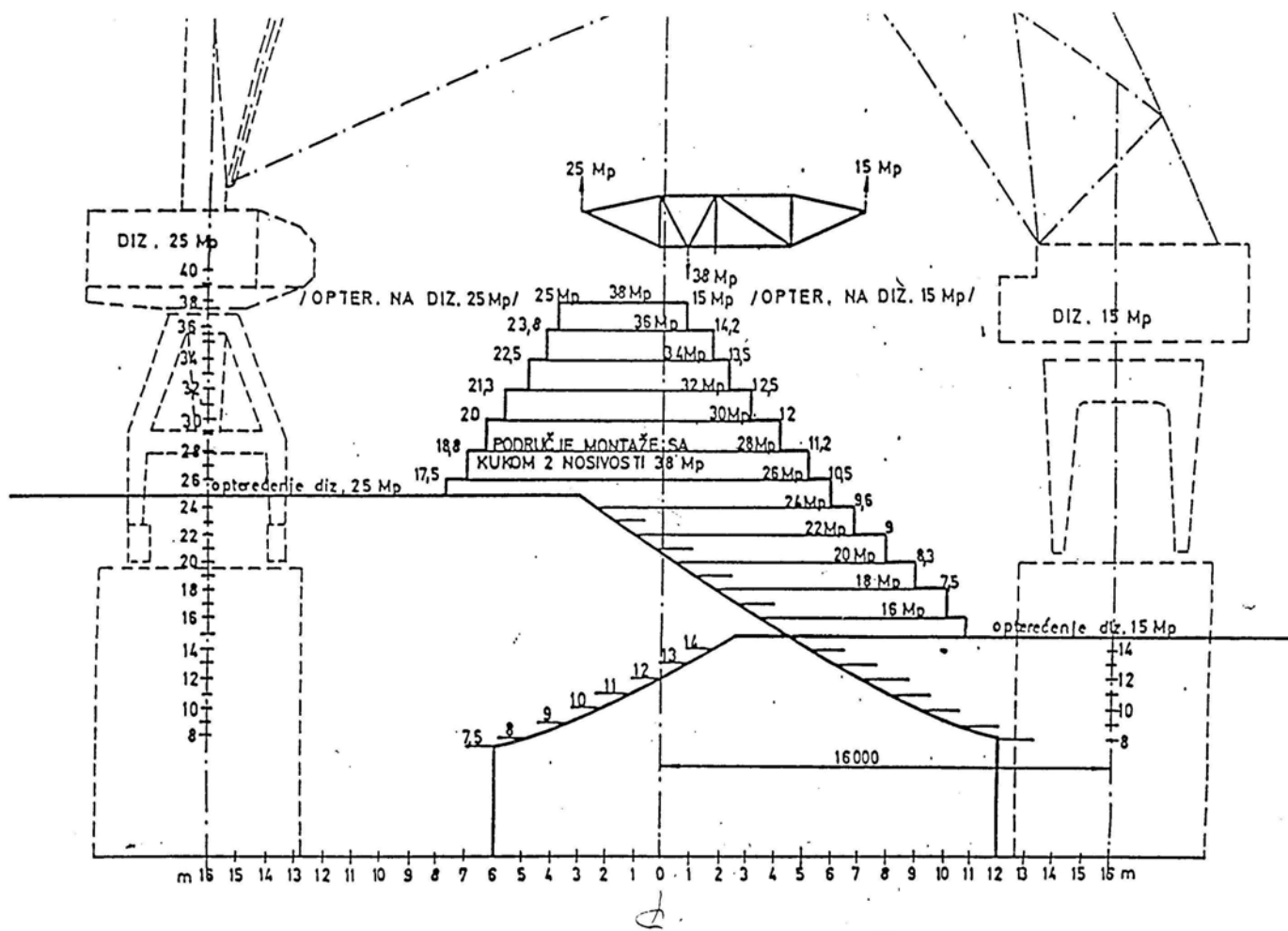
Slika 32 Dijagram kapaciteta dizalica na navozu br.2 kod režima pojedinačnog i tandem rada
