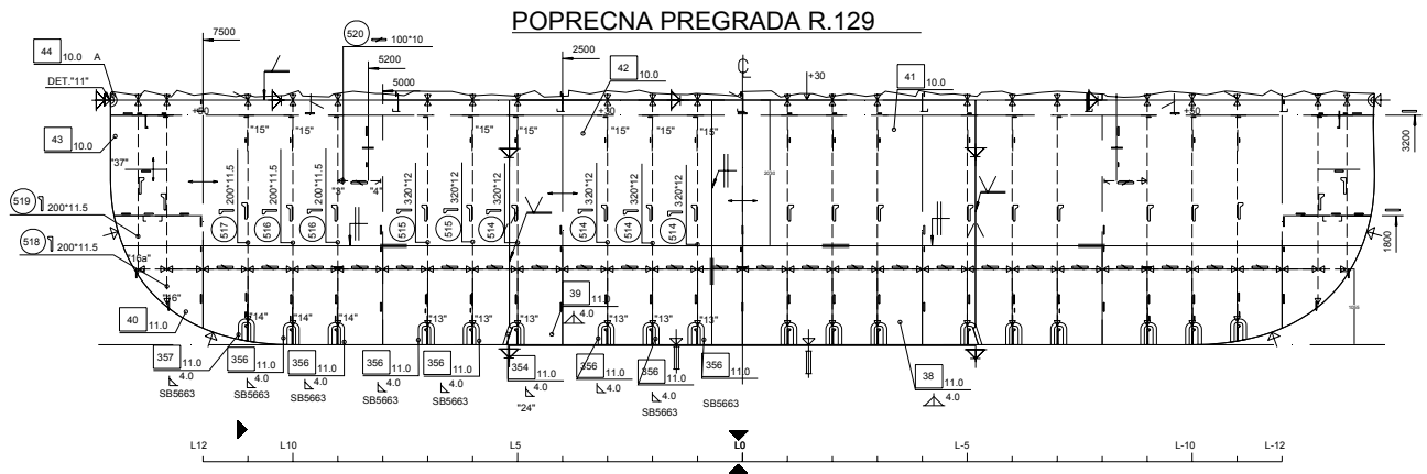
Slika 57 Poprečna pregrada na rebru R129
