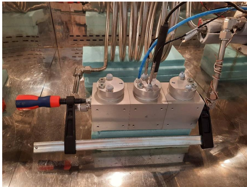
Slika 9. Mala komora unutar termostatisrane komore
