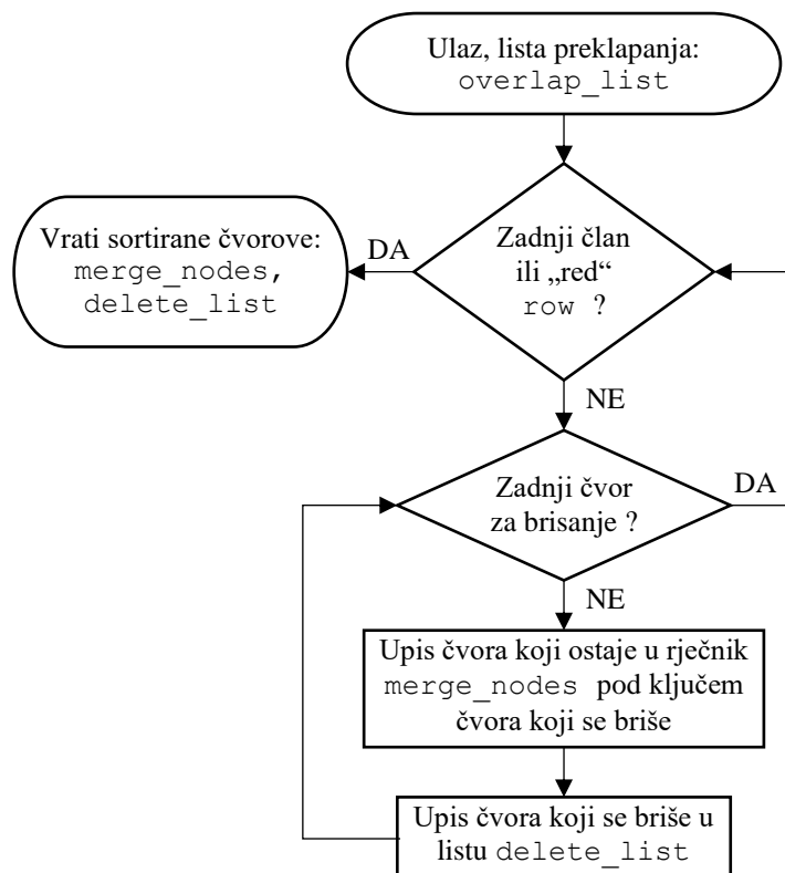
Slika 7.23 Dijagram toka metode sorted_coincident_nodes
