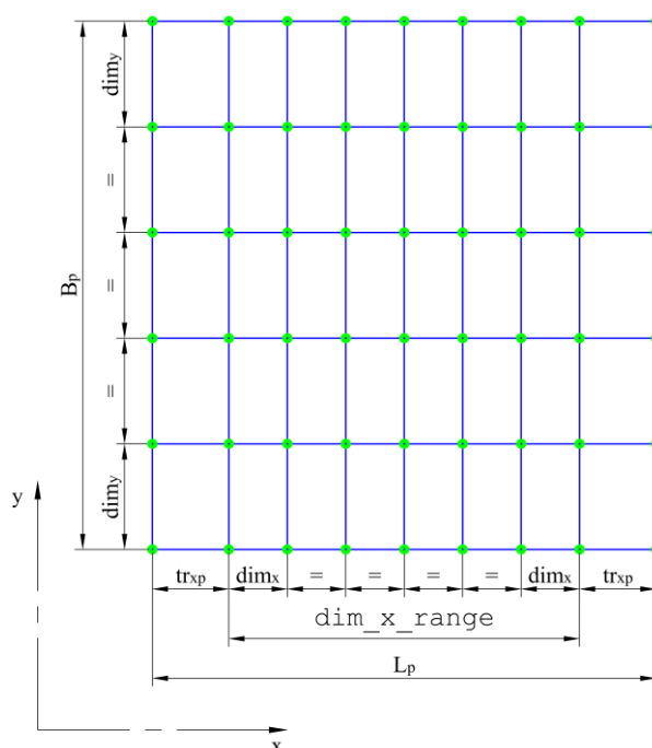
Slika 6.24 Broj konačnih elemenata osnovne mreže oplate
