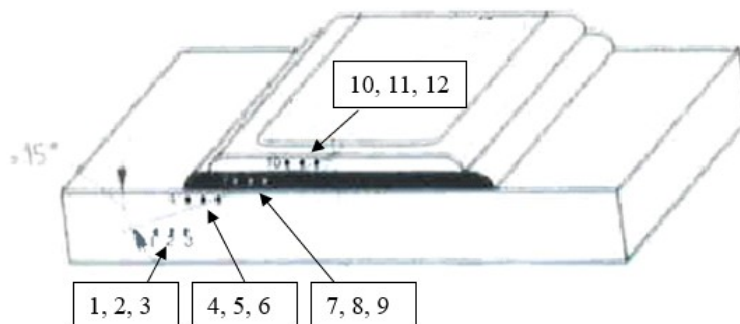
Slika 55 Raspored mjerenja tvrdoće HV10 na uzorku
