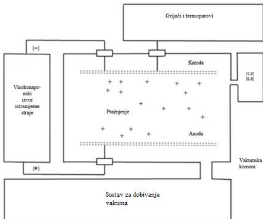
Slika 12. Shematski prikaz plazma nitriranja [7]
