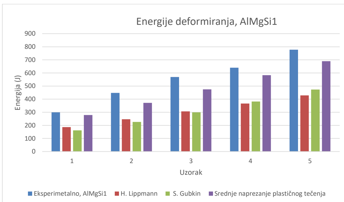
Slika 35. Grafički prikaz energija deformiranja prilikom sabijanja hidrauličnom prešom, legura AlMgSi1
