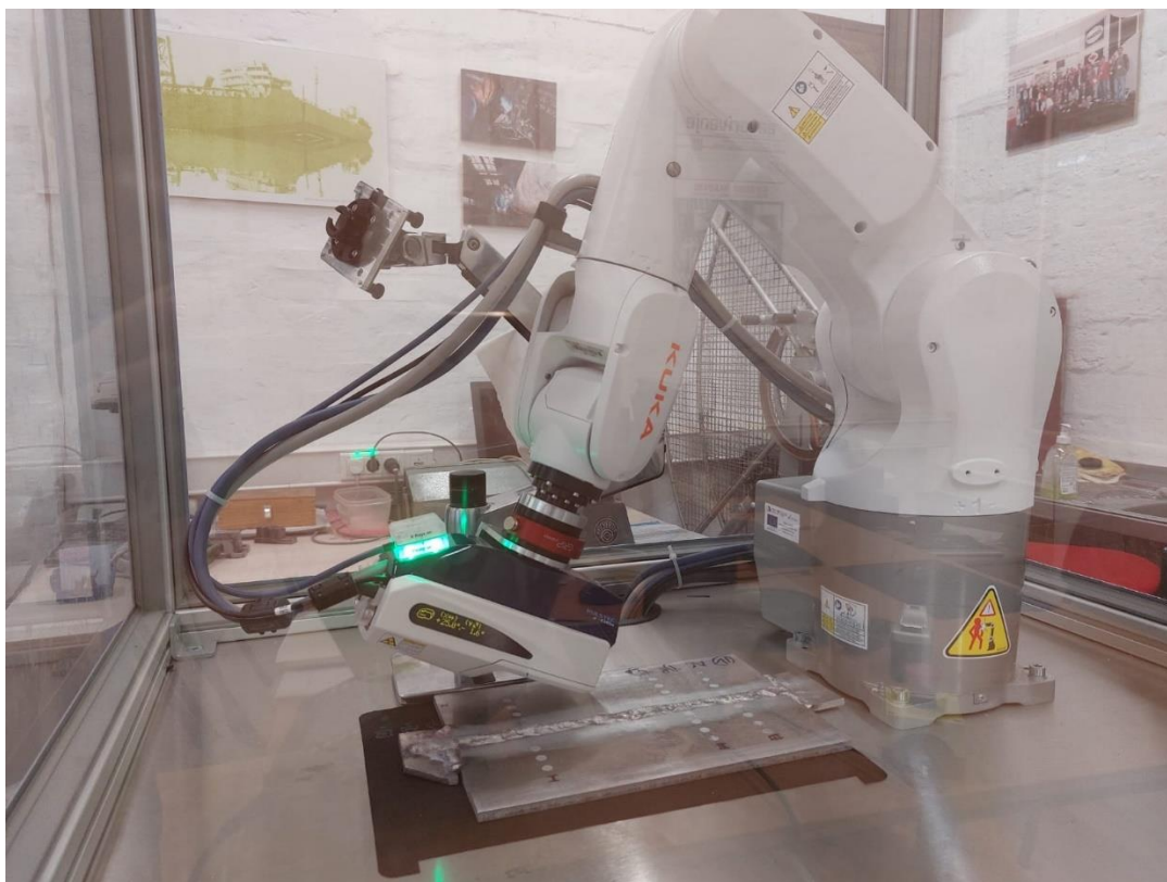
Slika 44. Pulstec \mu -X360s sa robotskom rukom marke Kuka
