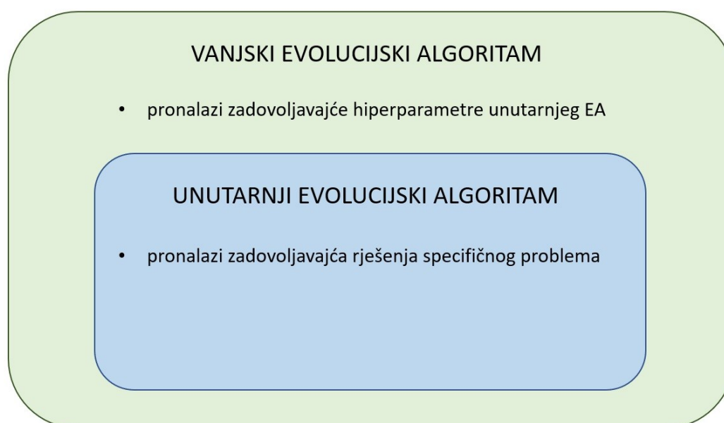
Slika 33. Struktura dubokih evolucijskih algoritama
