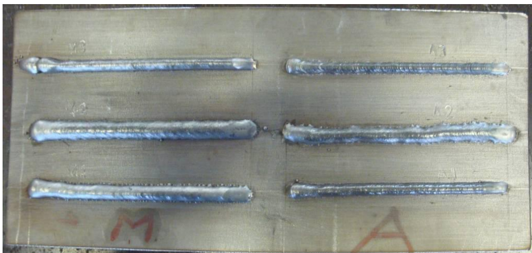
Slika 14. Navareni uzorci.
