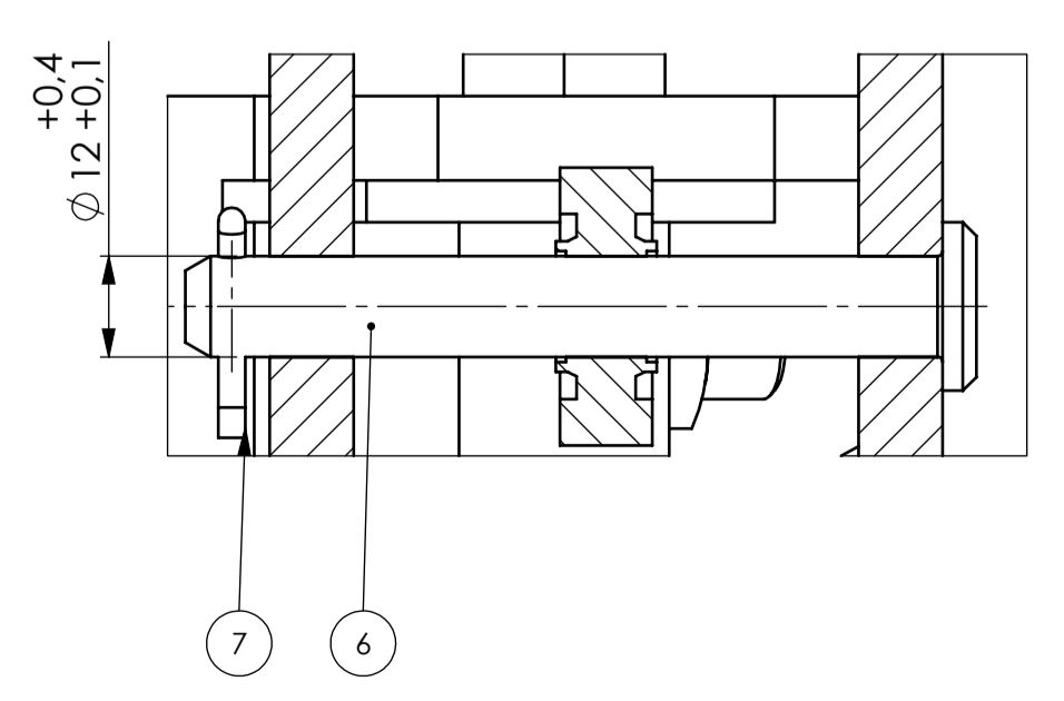
B-B (1 : 1)
