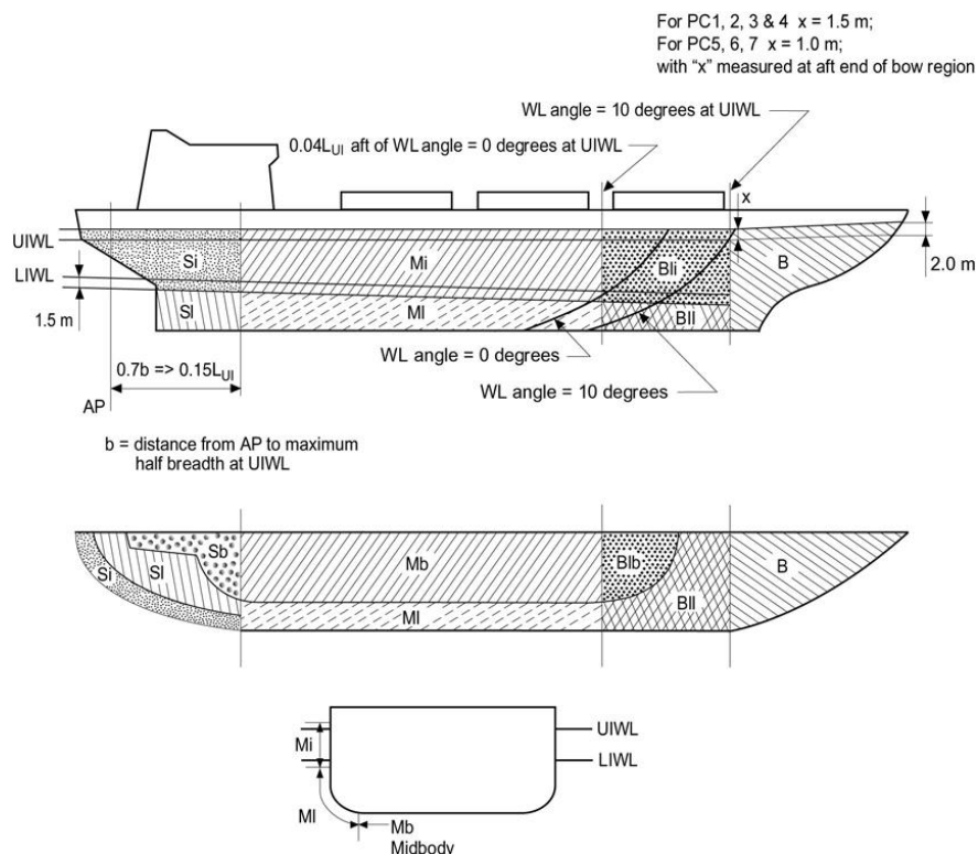
Slika 6. Raspored zona [3]
