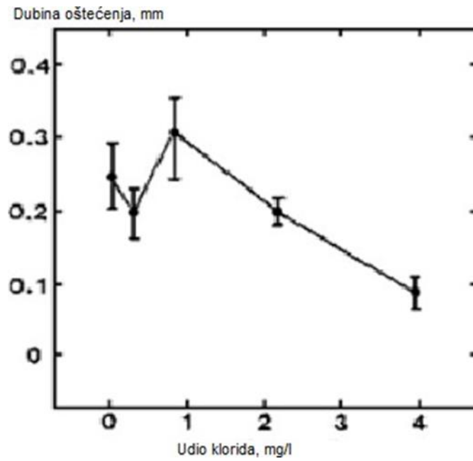
Slika 16. Dubina korozijskog oštećenja ovisno u udjelu klorida za 70/30 Cu – Ni leguru pri brzini strujanja morske vode od 9 m/s [12]
