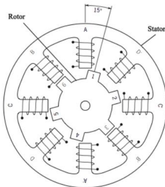
Slika 10. Koračni motor 3
