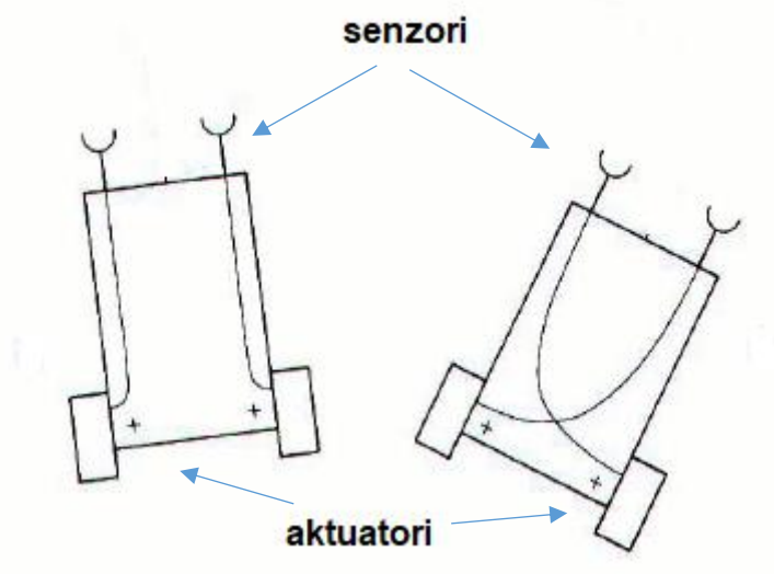
Slika 1. Braitenbergova vozila [2]
