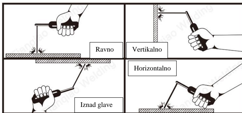
Slika 2: Položaji zavarivanja [3]
