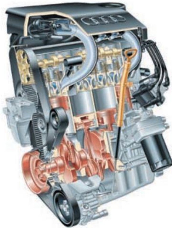
Slika 3.2. Presjek motora [14]
