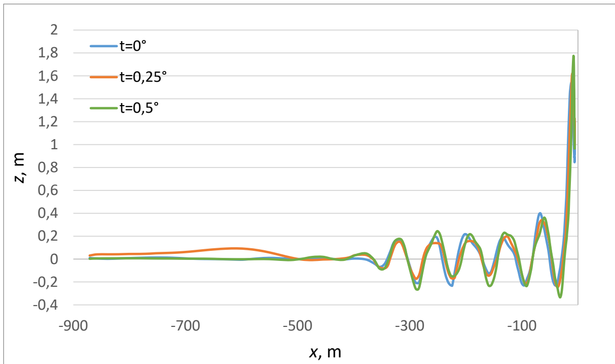
Slika 42. Usporedba valnih elevacija iza krme broda za ravnu vodnu liniju i pretegu u ravnini y=0 m
