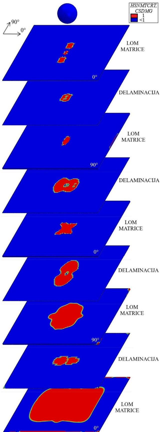
Slika 26. Aksonometrijski prikaz oštećenja matrice ( HSNMTCRT ) i delaminacija za laminat L2 - KP
