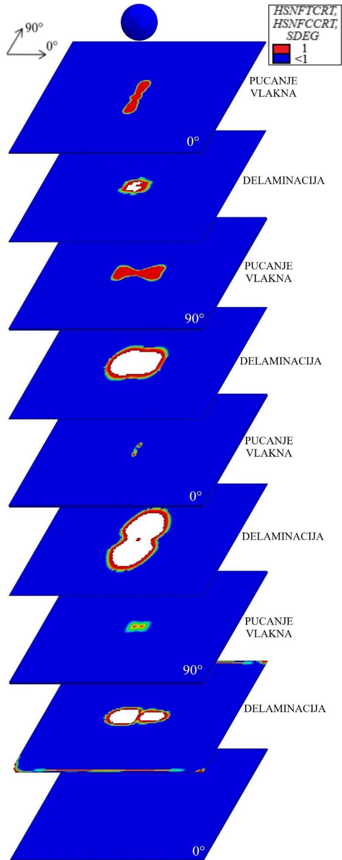
Slika 41. Aksonometrijski prikaz oštećenja vlakna i delaminacija za laminat L2 – KE
