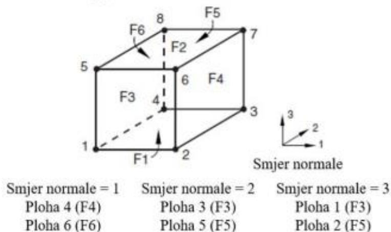
Slika 16. Mogući smjerovi normale SC8R konačnog elementa [26]
