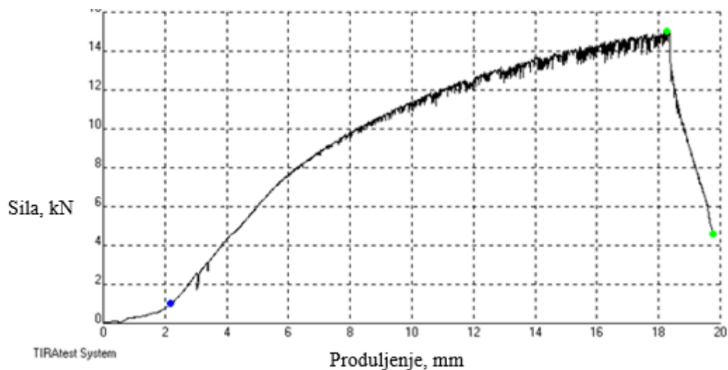
Slika 45. Dijagram sila-produljenje za uzorak 1b DC zavarenog spoja
