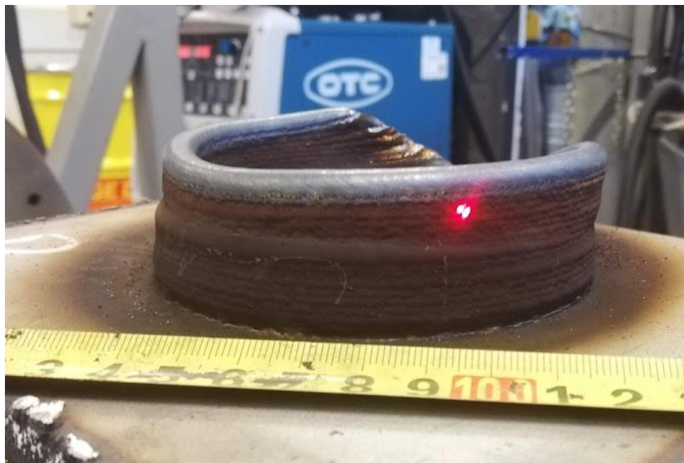
Slika 27. Uzorak D nakon zavarivanja
