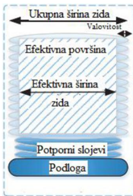
Slika 2. Shematski prikaz zida izrađen WAAM postupkom [5]
