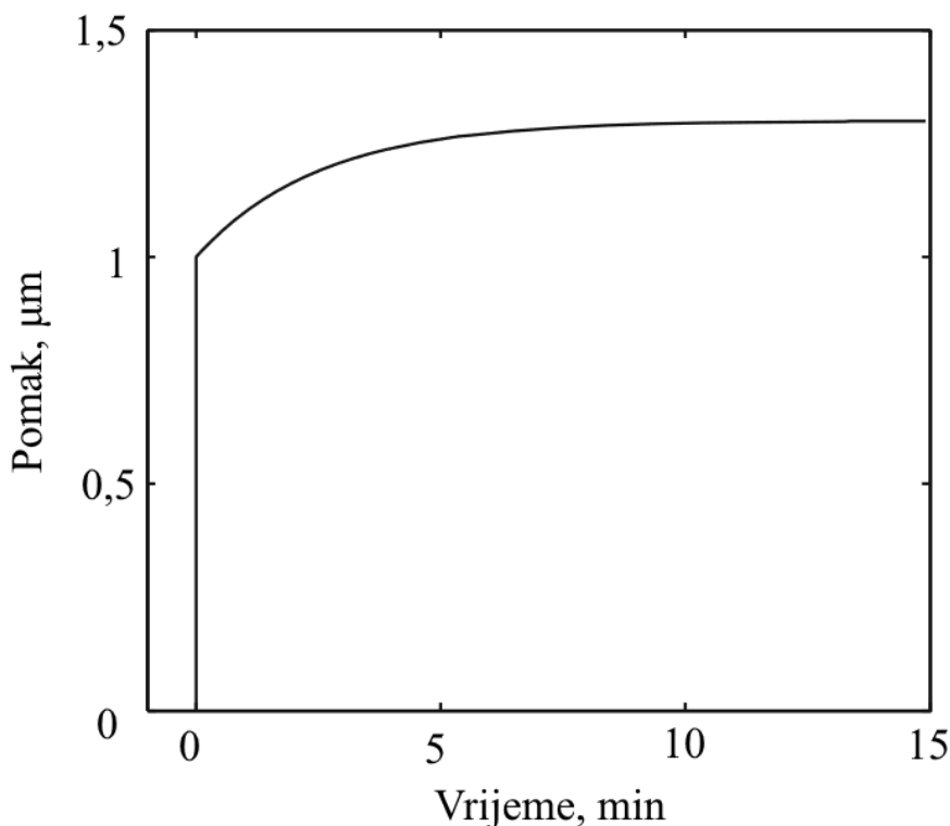
Slika 11. Prikaz puzanja (creep) kod piezoelementa [23]
