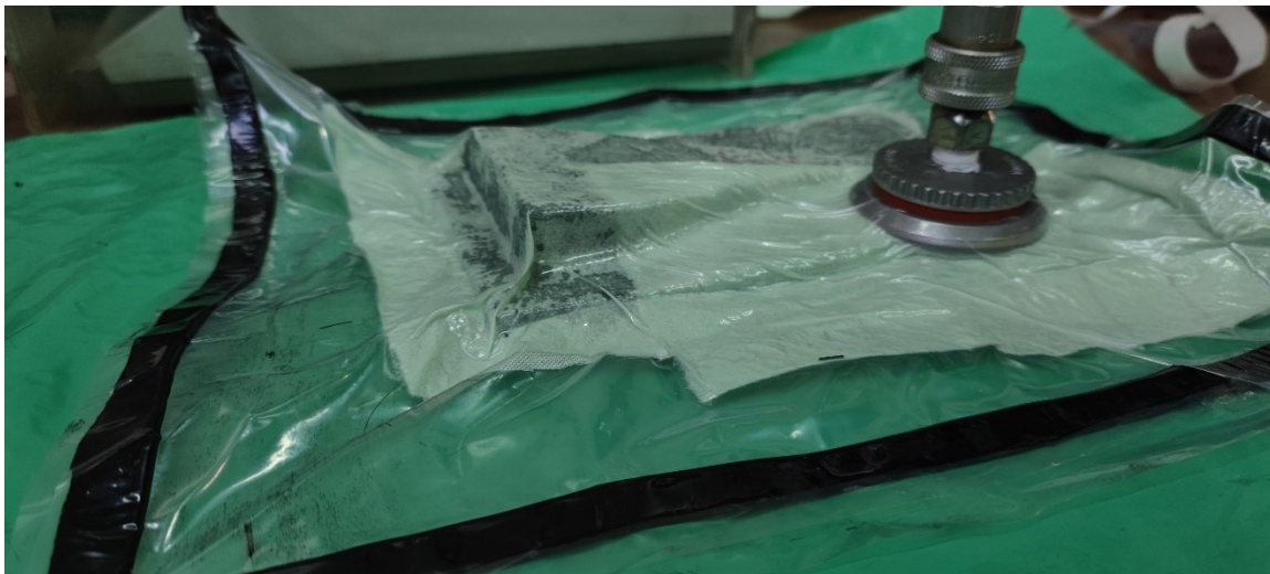
Slika 7.12. Istiskivanje zaostalog zraka u kompozitnom materijalu pomoću podtlačne pumpe
